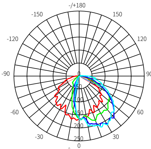
E2 EW 15W Empower
